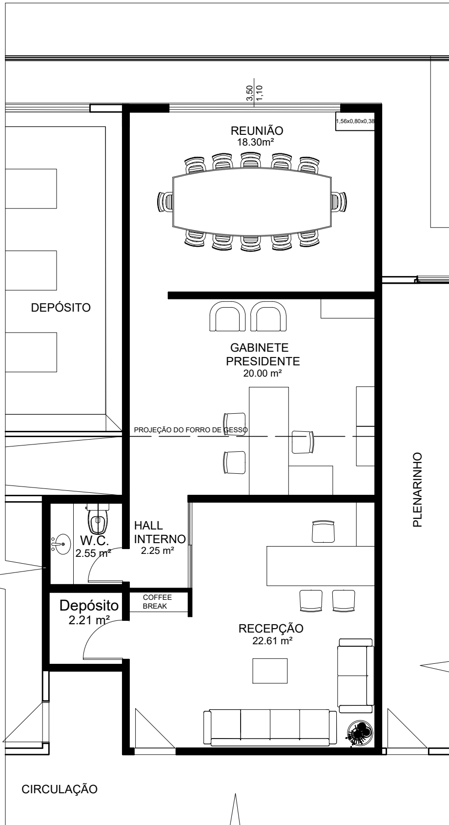
PLANTA BAIXA - TERREO (LAYOUT) ESCALA: 1 / 75
