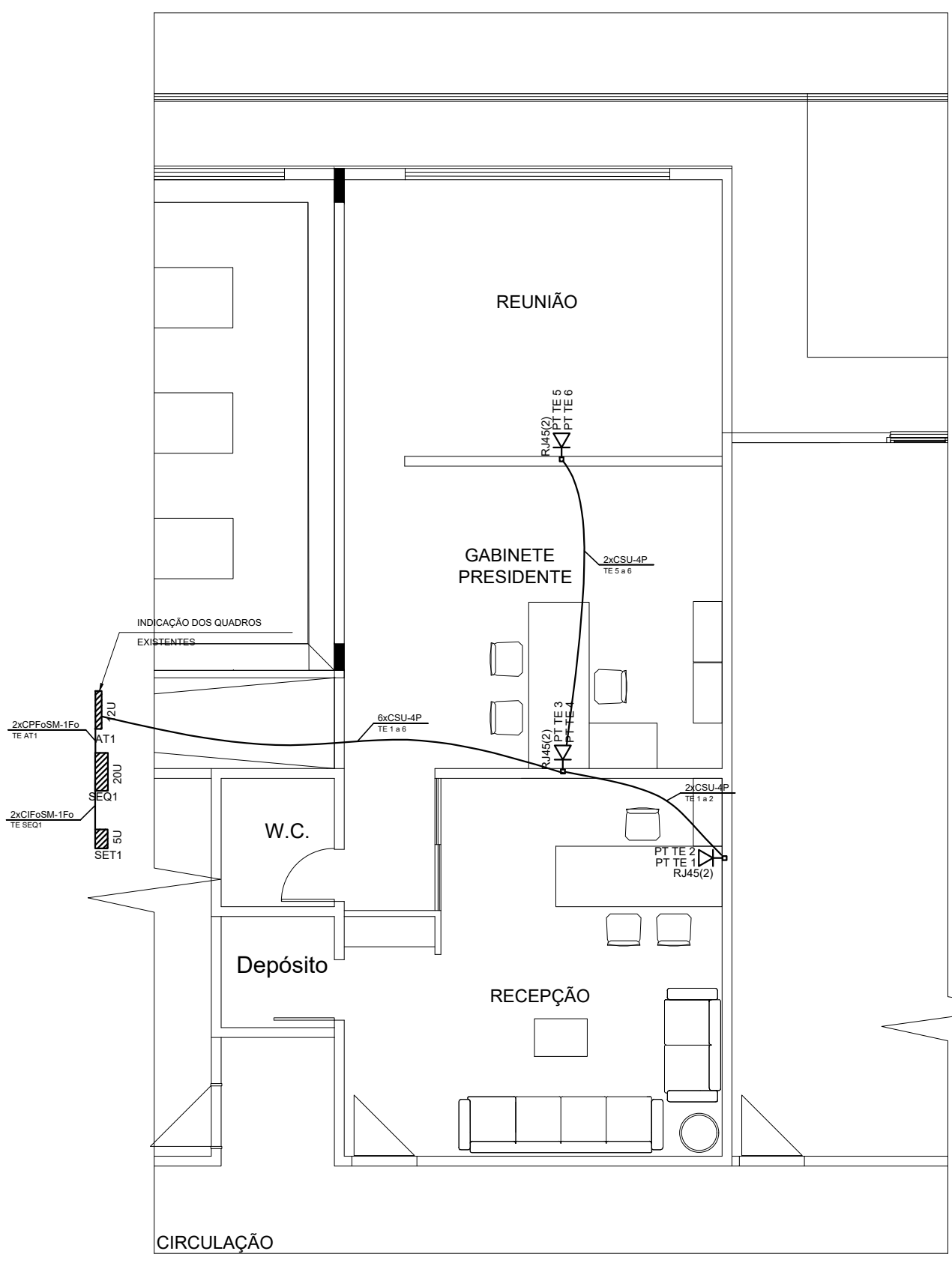
PLANTA BAIXA - TERREO (LAYOUT) ESCALA: 1 / 75
